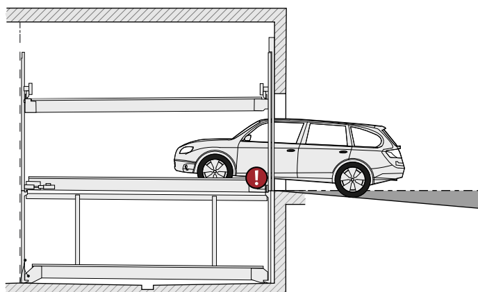
макс. угол подъема 5%
