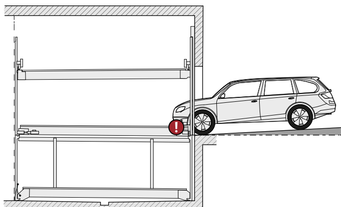
макс. угол съезда 3%
